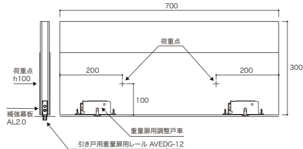
レール・戸車側面詳細
