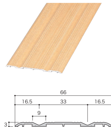
ウイングレール66W (66mm×3mm) 芯々33mm
