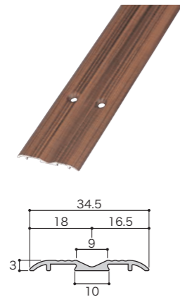
ウイングレール35S (35mm×3mm)
