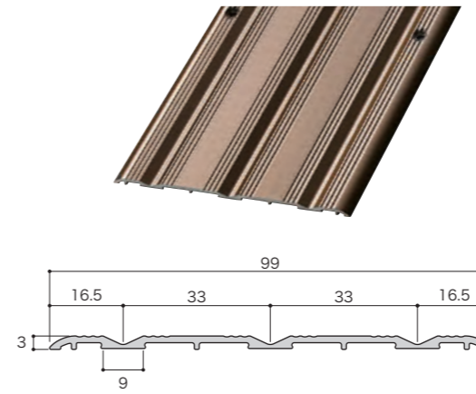
ウイングレール99T (99mm×3mm) 芯々33mm
