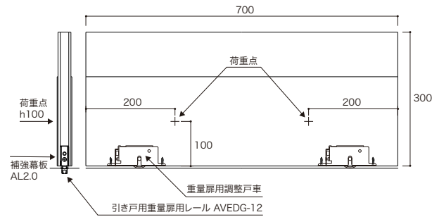
レール・戸車側面詳細
