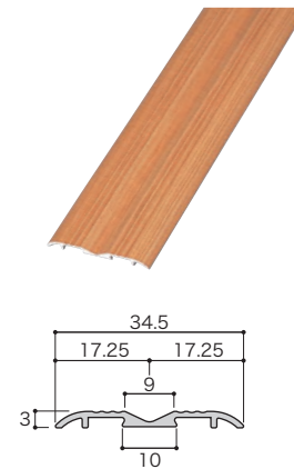
ウイングレール35SC (35mm×3mm)
