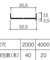
ドアエッジ (主に丁番取付用) 30B4 (旧 B-30-4) ● ステンカラー 有 抗菌
