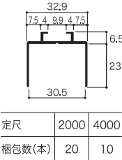
壁面取付エッジ 30B2M (旧 B-30-2N) ● ステンカラー 有 抗菌
