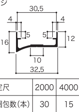
グレビティヒンジ用召合せエッジ 30B7 (旧 BR-30-7N) ● ステンカラー 有 抗菌
