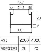
パネルジョイント 30B9 (旧 B-30-6) ● ステンカラー 有 抗菌
