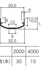
グレビティヒンジ用ドアエッジ 30B6 (旧 B-30-6) ● ステンカラー 有 抗菌
