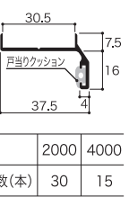
召合せエッジ 戸当りクッション付 30B1WD (旧 B-30-1DN) ● ステンカラー 有 抗菌
