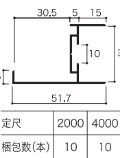
コーナーエッジ 30B5 (旧 B-30-5) ● ステンカラー 有 抗菌
