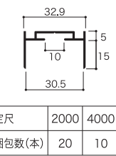
壁面取付エッジ 30B2 (旧 B-30-2) ● ステンカラー 有 抗菌
