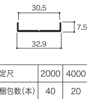
ドアエッジ 30B3 (旧 B-30-3) ● ステンカラー 有 抗菌
