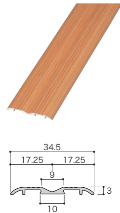
ウイングレール35SC (35mm×3mm)
