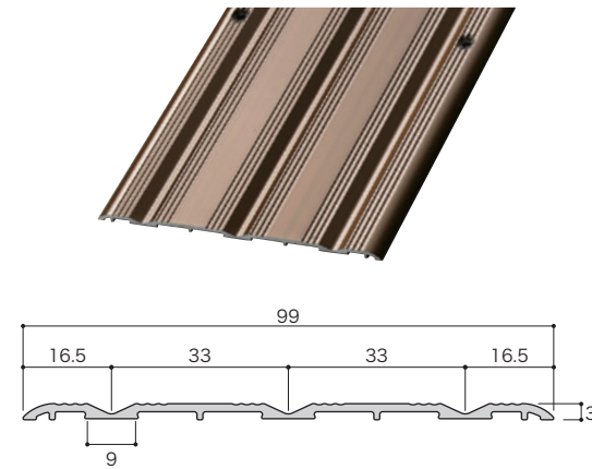
ウイングレール99T (99mm×3mm) 芯々33mm
